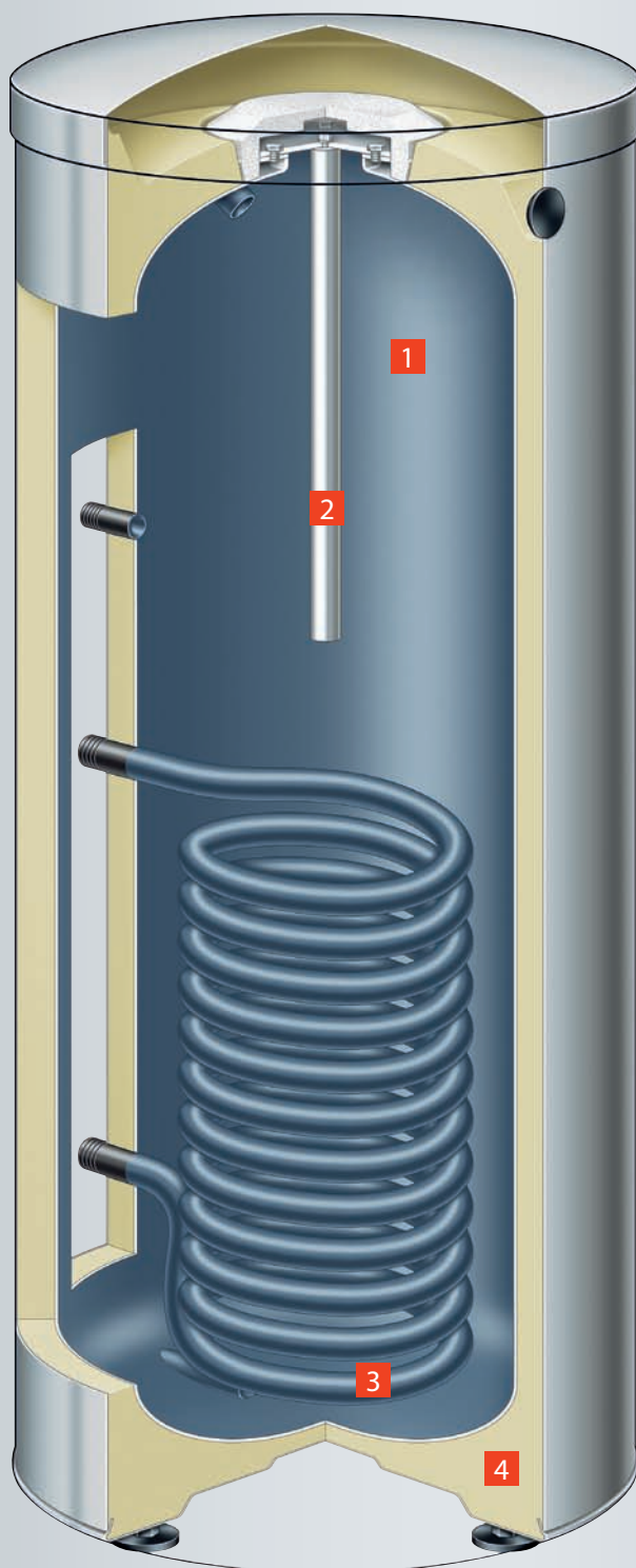
Vitocell 100-V (тип CVA, 160 литров)
