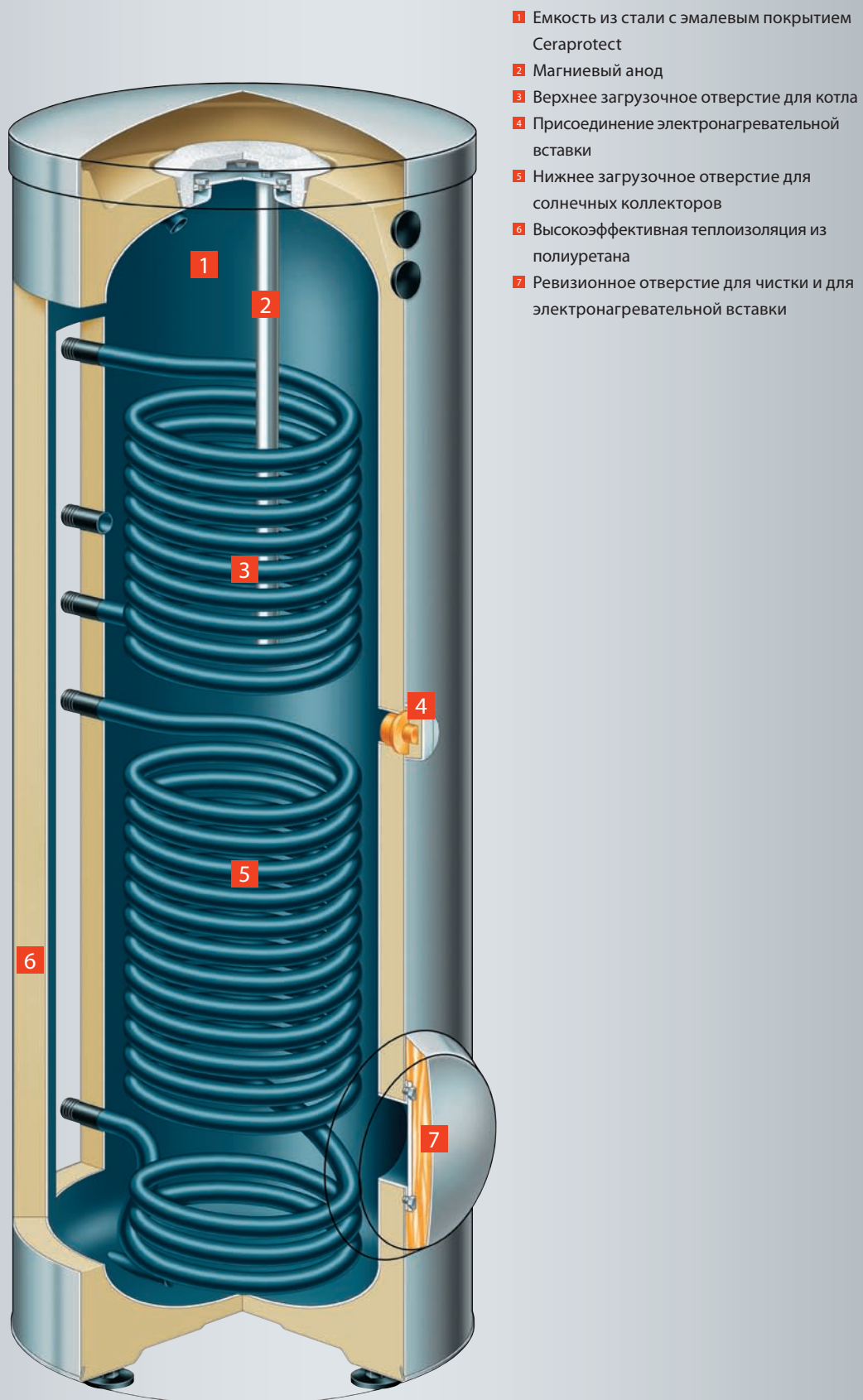
Vitocell 100-B (тип CVB)
