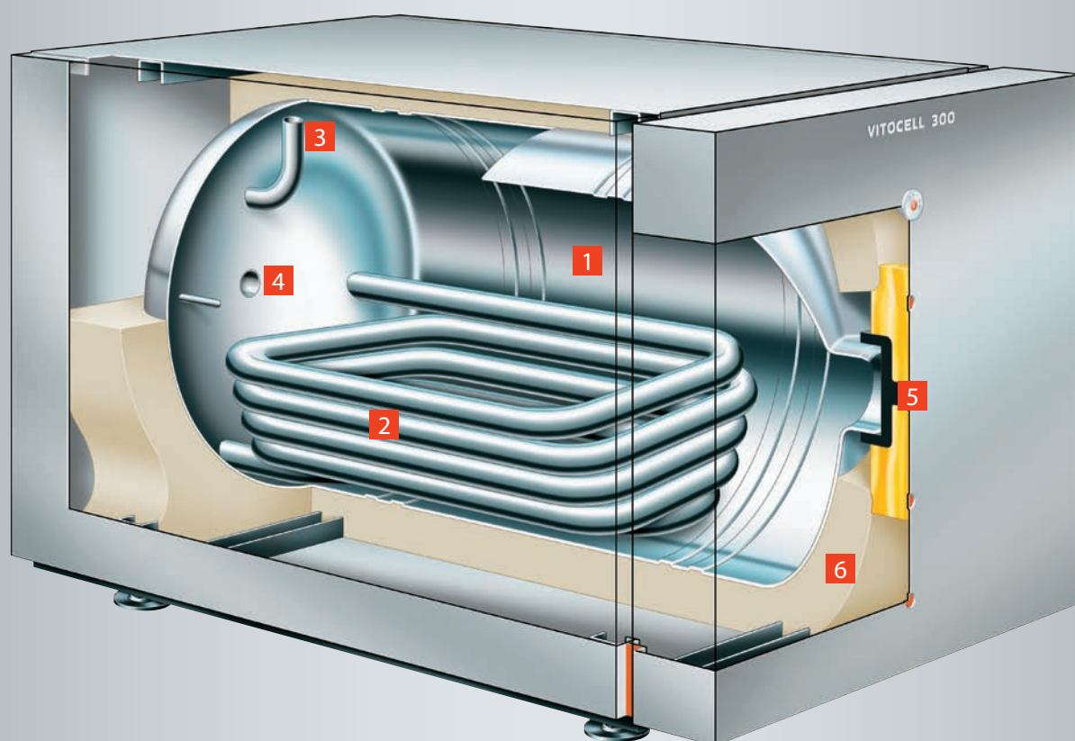
Vitocell 300-H (тип ЕНА)
