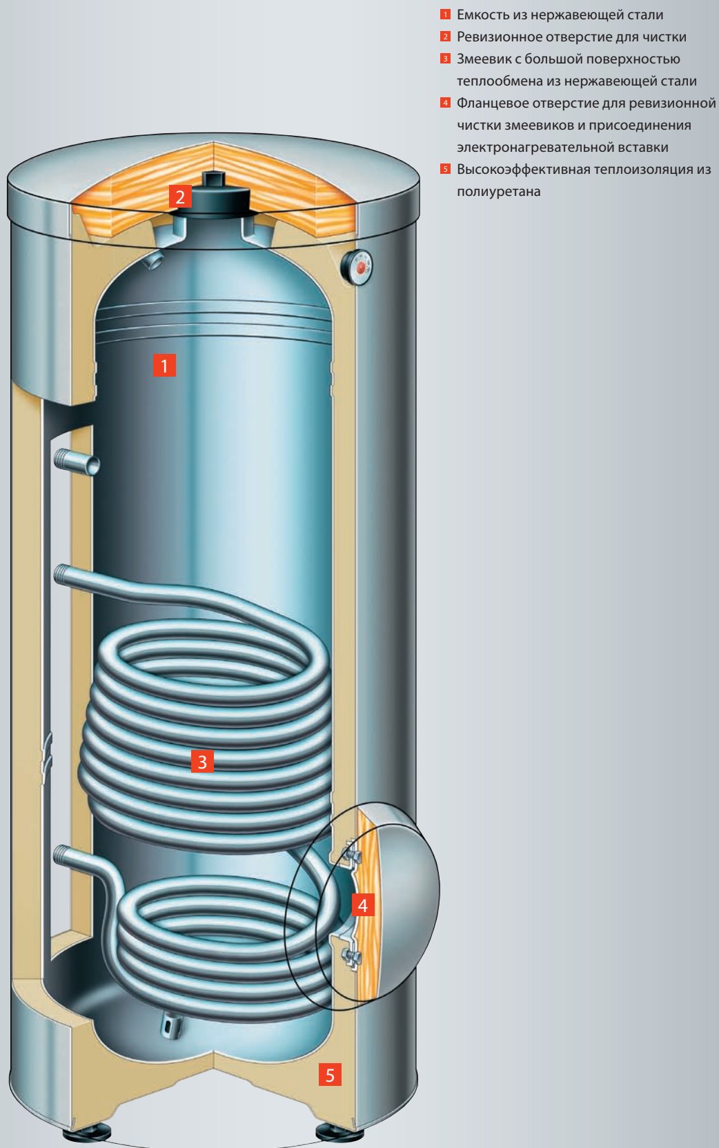
Vitocell 300-V (тип EVI, 200 и 300 литров с фланцевым отверстием)
