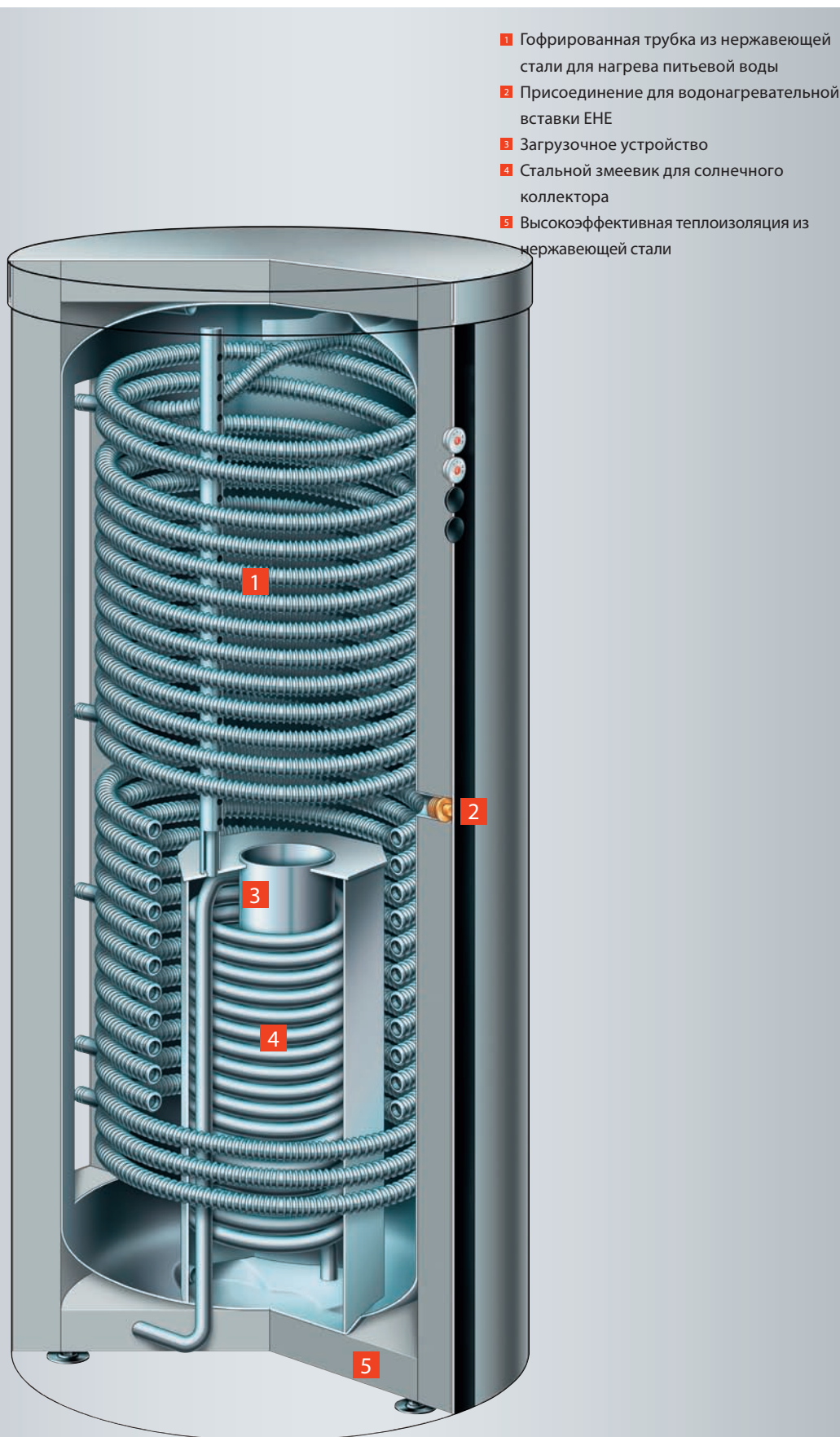
Vitocell 360-M (тип SVSA)
